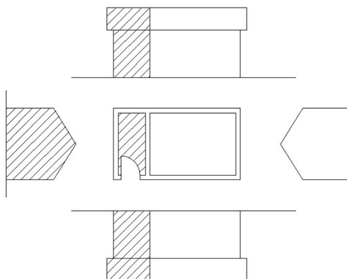
schema 2: tetto a due falde
