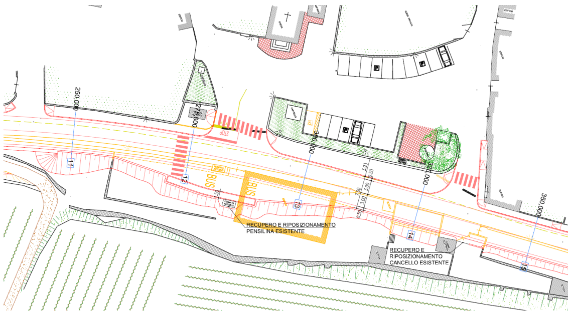
Estratto della tavola di raffronto (opera S-841)
